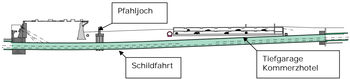
Länasschnitt Vortrieb Ost
